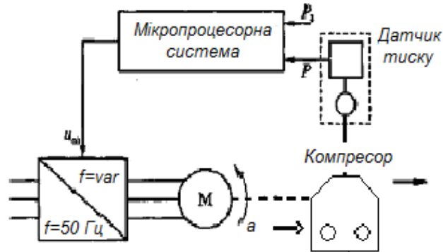
Рисунок 3 – Мікропроцесорна система управління
