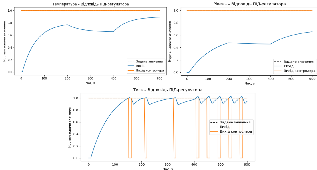
Рисунок 4 – Результати моделювання проекрованої КСУ
