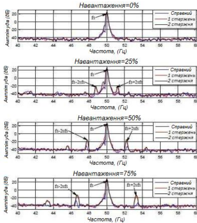
Рисунок 5 – Спектри струму асинхронного двигуна при різних навантаженнях
