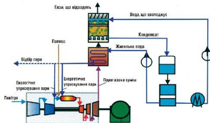
Рисунок 2 - Принципова схема ПЕА
