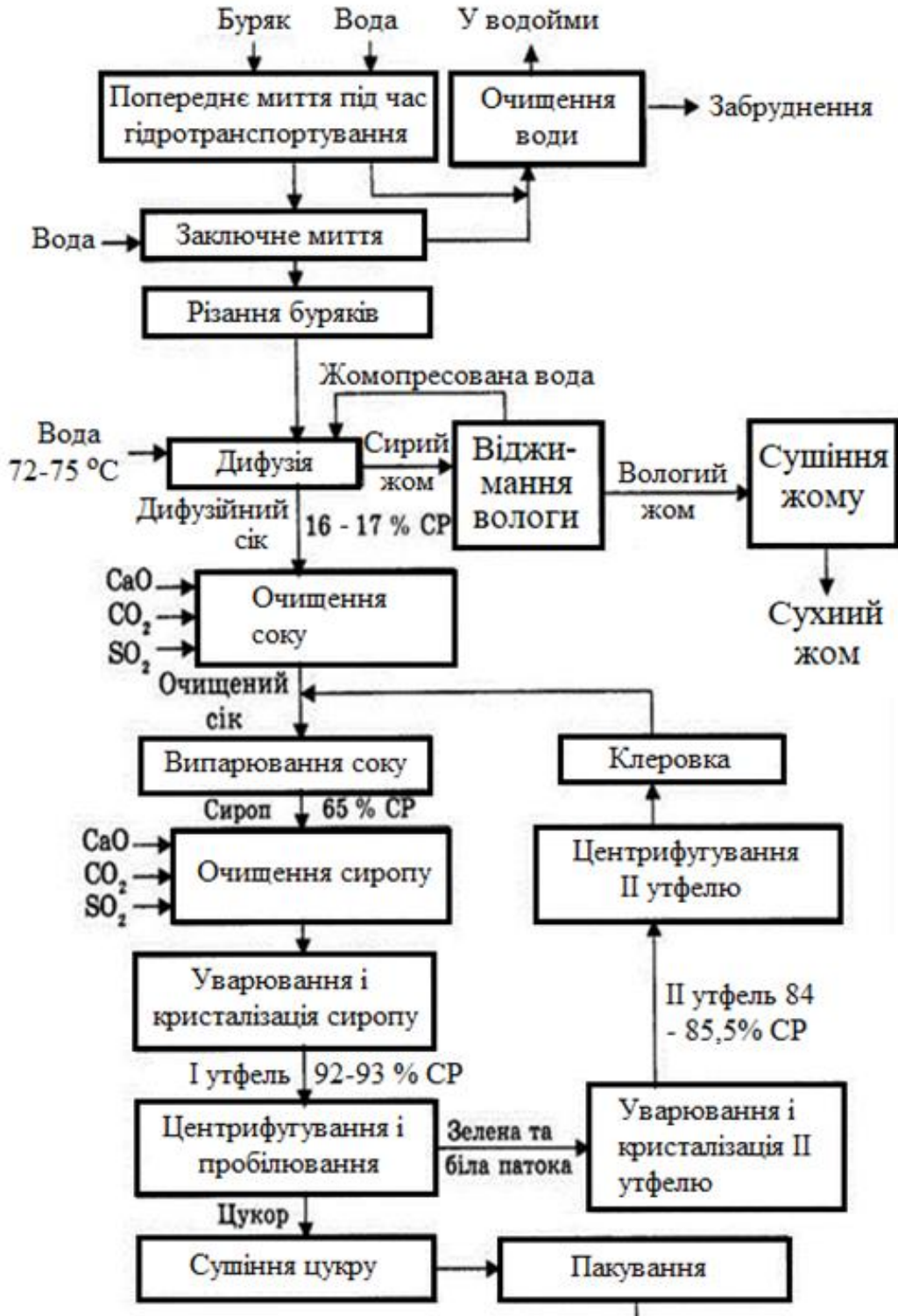
Рисунок 1 - Принципова технологічна схема виробництва цукру з буряку
