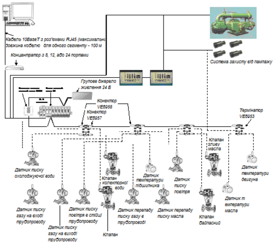
Рисунок 5 – Структурна схема САУ компресора
