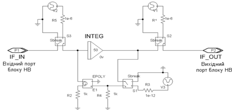
Рисунок 2 – Схема моделі блока реалізації способу визначення інтегралу функції за період
