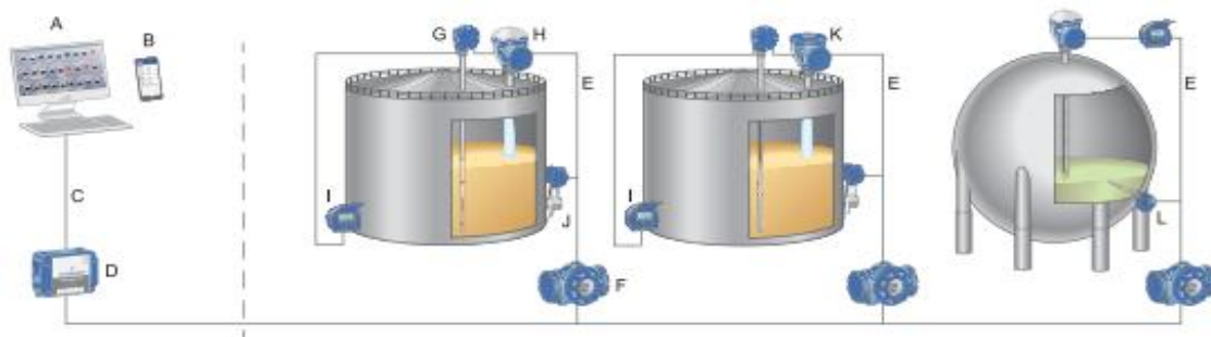
Рисунок 2 – Структура АСУ
